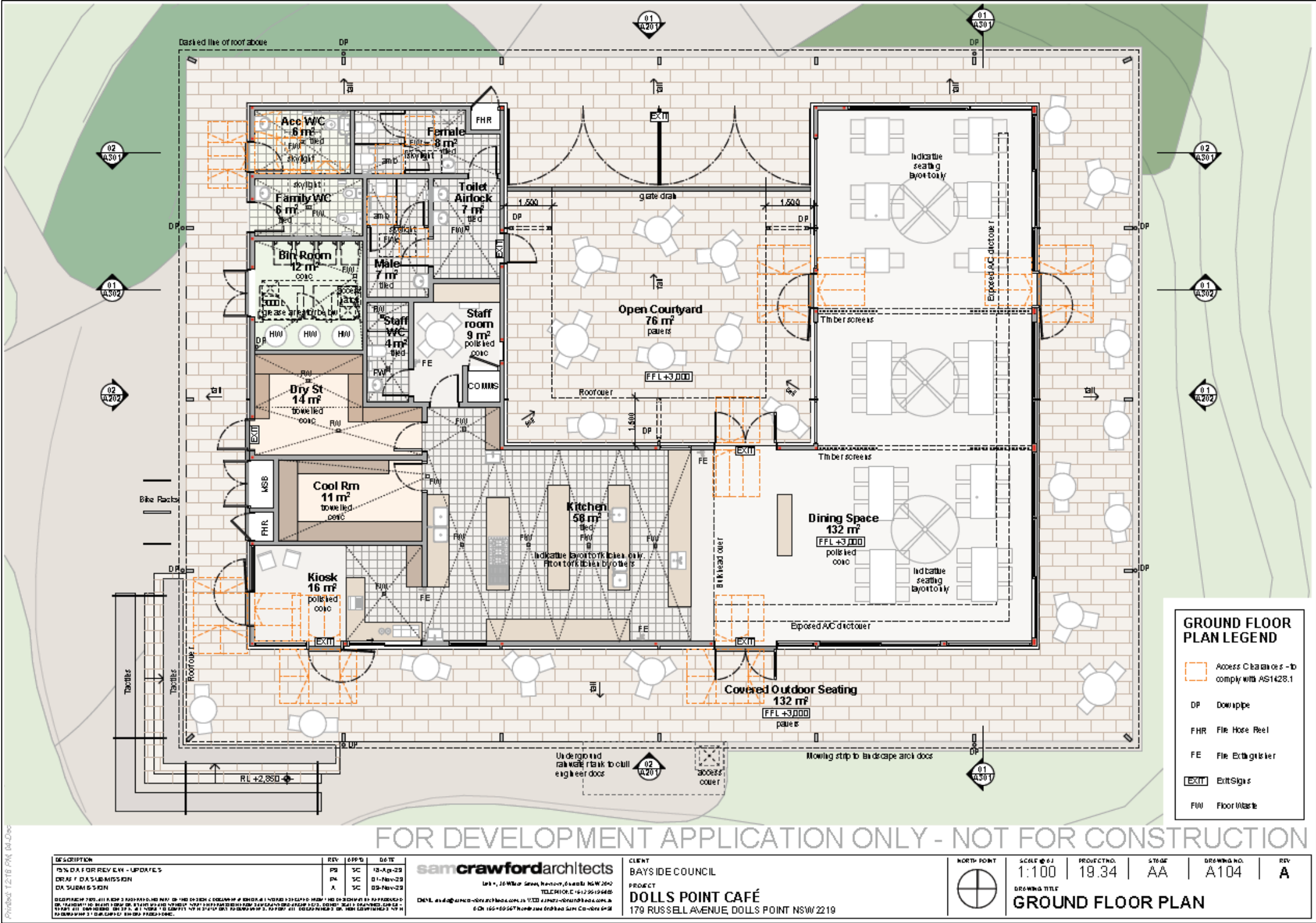
Item 1.1.2: Site Plan
